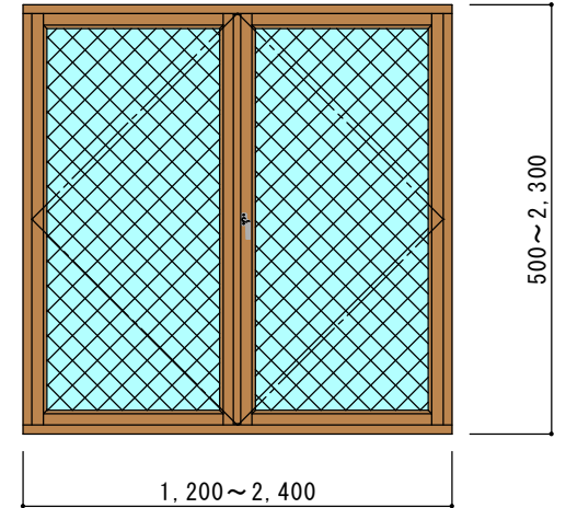
両開き窓 (WSH56) (認定番号: EB-0076) 単板 (PW6.8)
