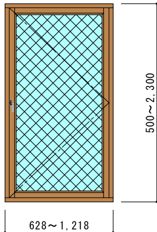
片開き窓 (SSH56) (認定番号: EB-0076) 単板 (PW6.8)
