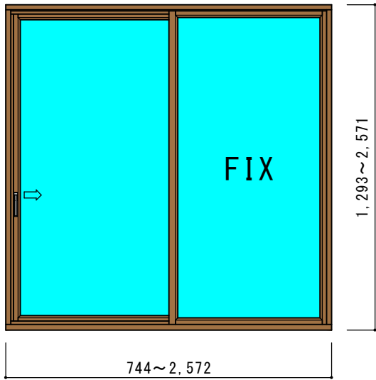
FIX付エコスライド窓 EB-2380 遮熱高断熱複層硝子 (Low-E5+AR16+結晶化4)
