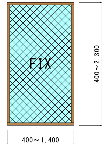
はめ殺し窓 (FIX56) (認定番号: EB-0034) ペア (PW6.8+A6+FL5)
