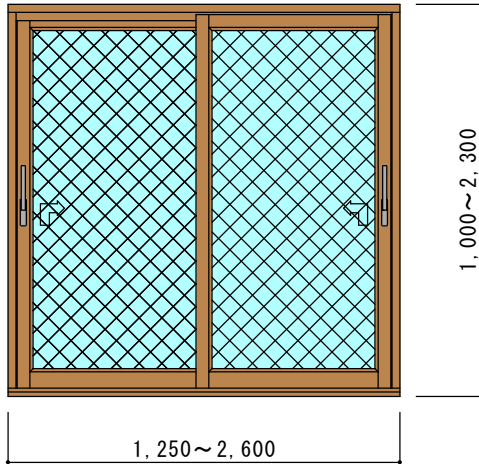
引き違い窓 (WHS56) (認定番号: EB-0090) 単板 (PW6.8)
