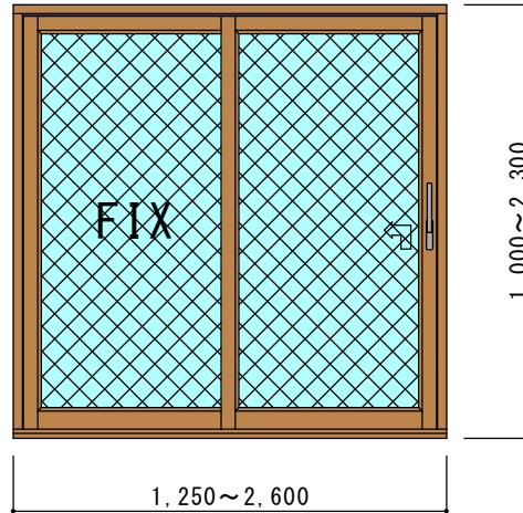
片引き窓 (SHS56) (認定番号: EB-0090) 単板 (PW6.8)
